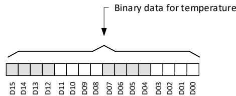
图 7-6. Temperature Sensor Data Definition
