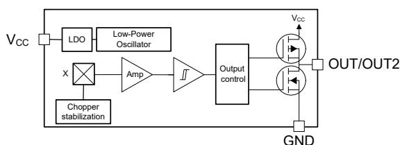
ブロック図 (プッシュプル)
