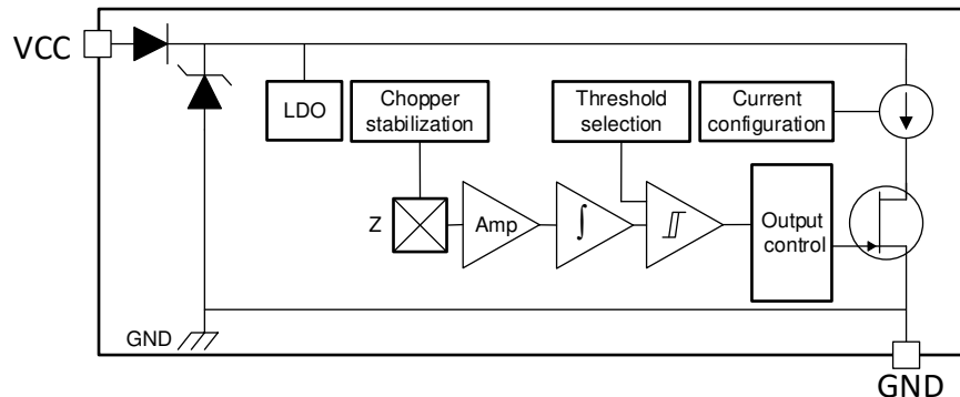
図 8-1. Block Diagram
