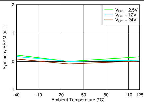
図 6-62. B_{SYM(Y)} vs Temperature
