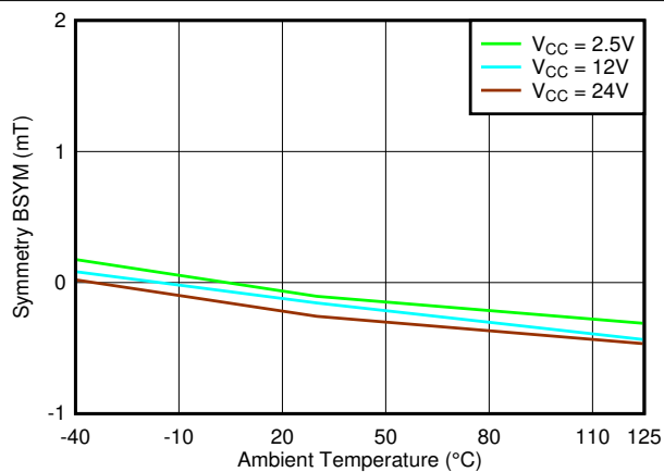
図 6-60. B_{SYM(X)} vs Temperature
