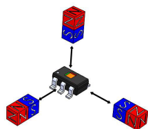
デバイス軸の極性
