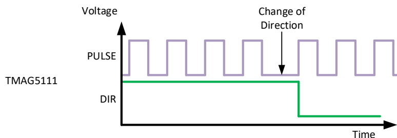
图 9-3. TMAG5111 Output Response
