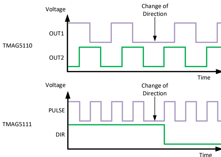
デバイス出力
