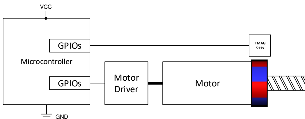
図 9-1. Incremental Encoding
