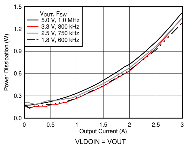
図 6-8. Power Dissipation
