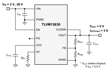
代表的な回路図
