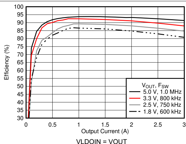
図 6-7. Efficiency
