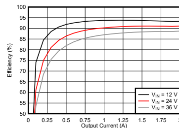
代表的な効率 ( V_{OUT} = 5V 、 f_{SW} = 1MHz )
