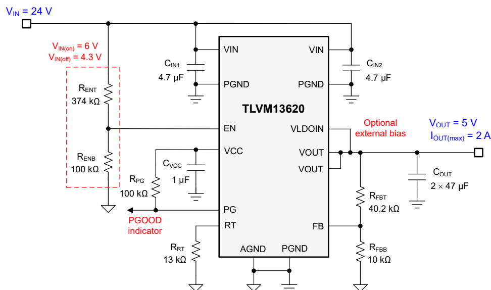
図 9-1. Circuit Schematic
