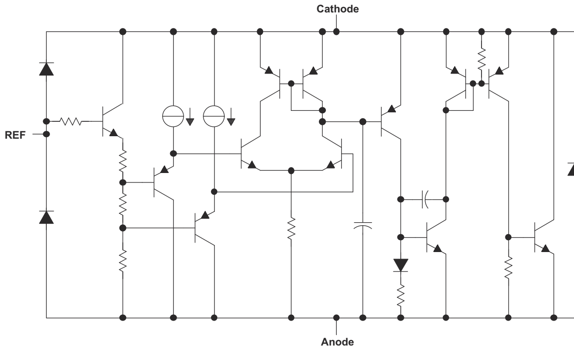
図 7-2. Detailed Schematic
