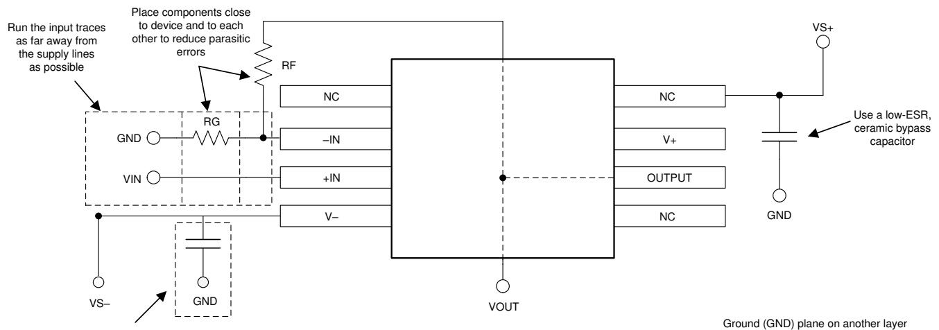
図 7-3. 回路図
