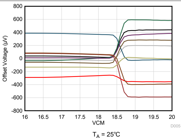
図 5-6. オフセット電圧と同相電圧との関係 (遷移領域)
