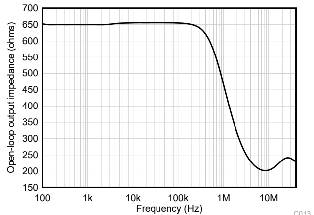
図 5-26. 開ループ出力インピーダンスと周波数との関係
