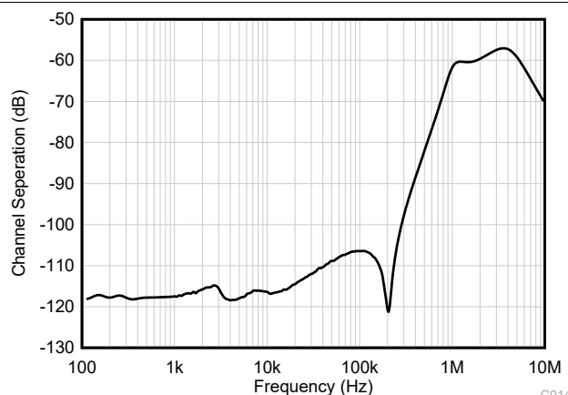
図 5-40. チャネル分離と周波数との関係
