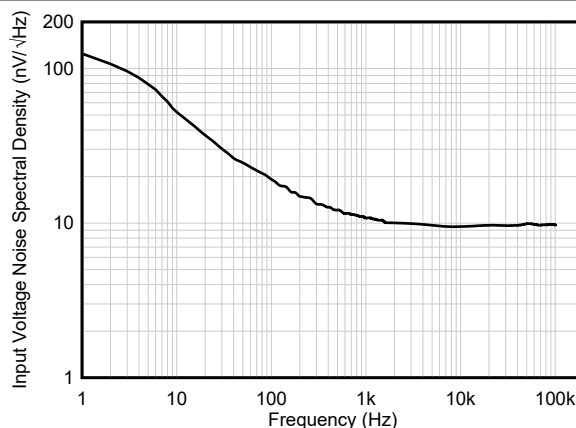
図 5-20. 入力電圧ノイズ・スペクトル密度と周波数との関係
