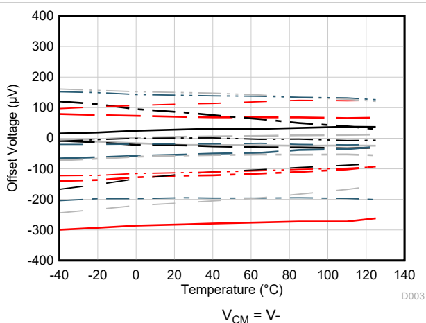
図 5-4. オフセット電圧と温度との関係
