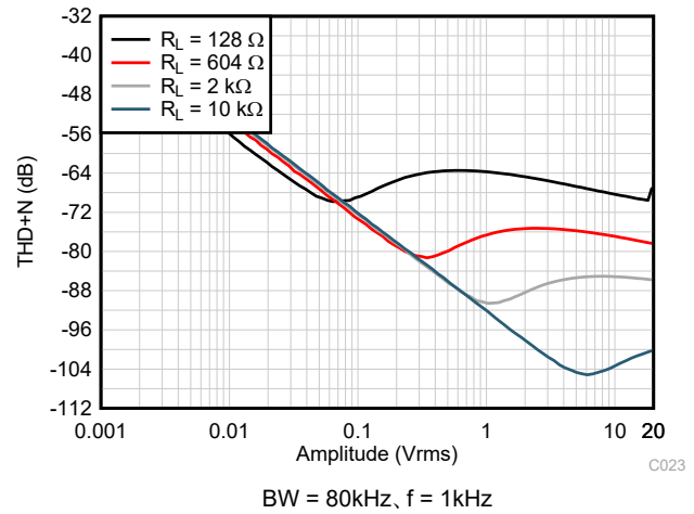
図 6-22. THD+N と出力振幅との関係
