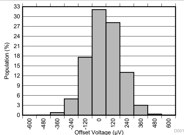
図 5-1. オフセット電圧の製造分布
