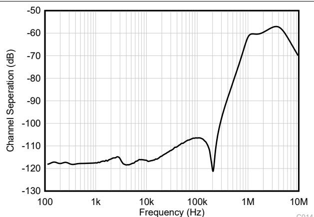
図 5-40. チャネル分離と周波数との関係
