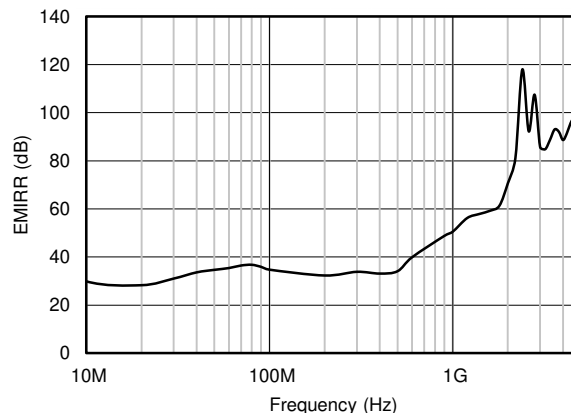
図 6-1. EMIRR Testing
