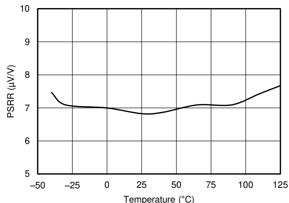
図 5-14. PSRR vs Temperature
