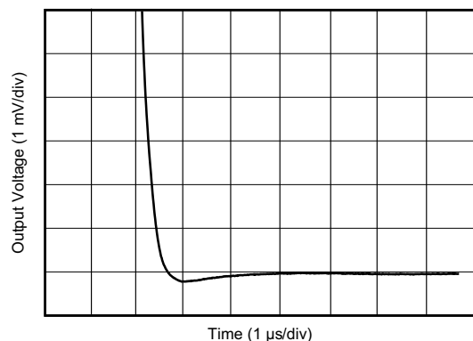
図 7-31. 大信号のセリング・タイム (負)
