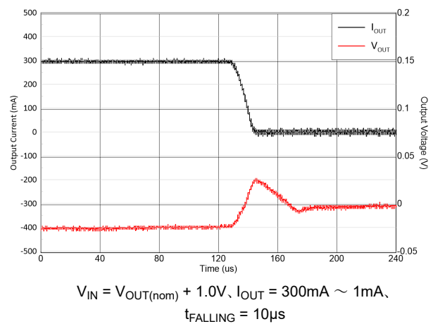
図 5-12. 負荷過渡
