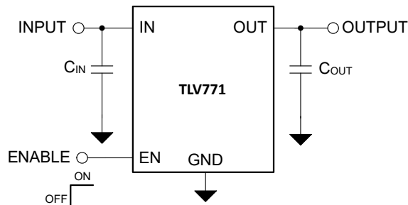
図 7-1. TLV771 の代表的なアプリケーション
