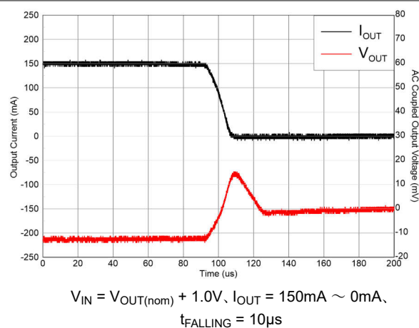
図 5-12. 負荷過渡
