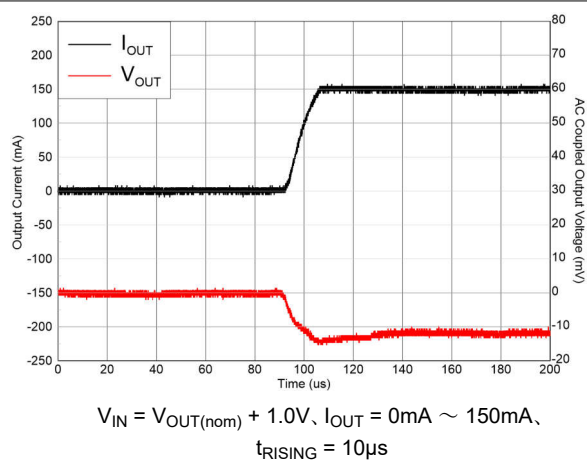
図 5-11. 負荷過渡
