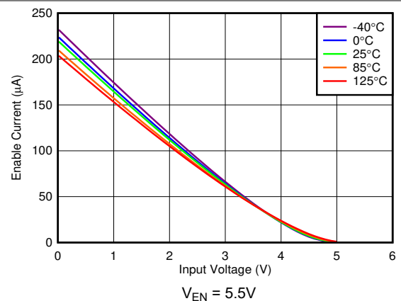
図 5-24. I_{EN} vs V_{IN}
