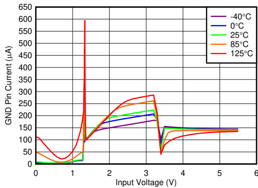
図 5-19. I_{GND} vs V_{IN}
