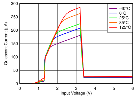
図 5-20. I_{GND} vs V_{IN}
