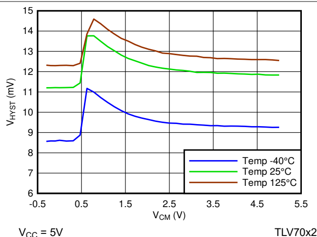
図 5-16. Hysteresis vs V_{CM}
