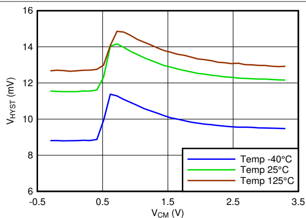
図 5-15. Hysteresis vs V_{CM}
