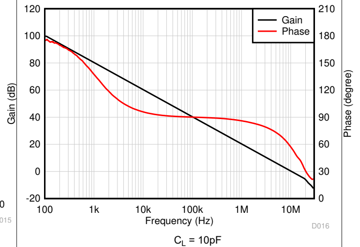
図 7-54. 開ループのゲインおよび位相と周波数との関係
