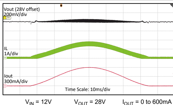
図 8-16. Load Sweep
