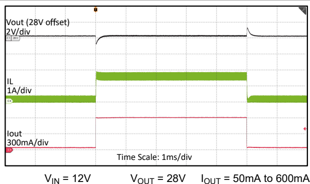
図 8-15. Load Transient
