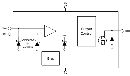
オープン ドレイン出力のブロック図
