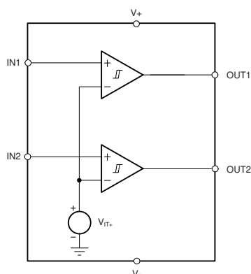
TLV4062-Q1 のブロック図
