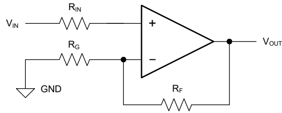
図 7-4. 回路図
