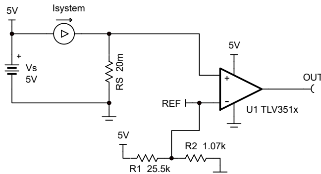
図 7-7. 電流検出
