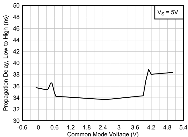
図 5-38. 伝搬遅延 - Low から High vs.5V でのコモンモード
