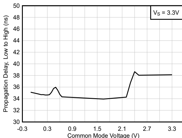
図 5-40. 伝搬遅延、"Low" から "High" と 3.3V でのコモンモードの関係
