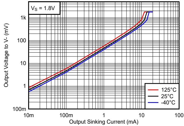
図 5-19. 出力電圧と 出力シンク電流の関係、1.8V
