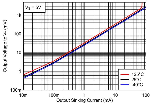
図 5-23. 出力電圧と 出力シンク電流の関係、5V
