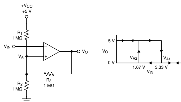
図 7-3. ヒステリシス付き反転構成の TLV321x
