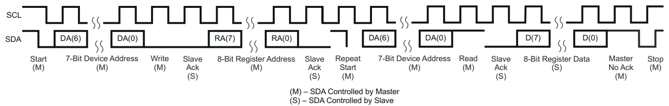
図 7-15. I 2 C Read
