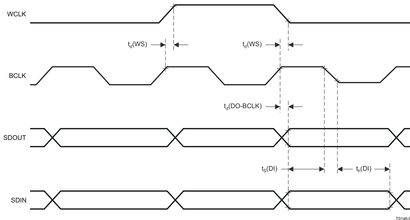
図 6-3. DSP Timing in Master Mode
