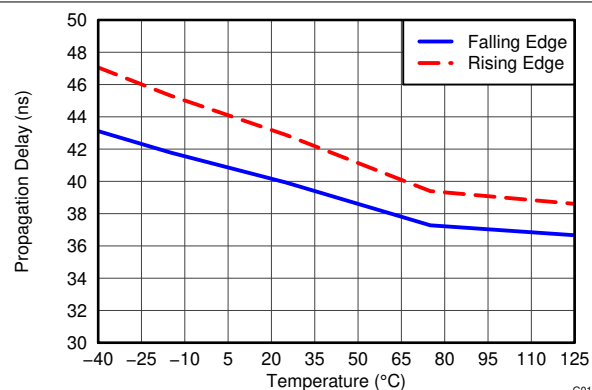
図 6-20. 伝播遅延と温度との関係
