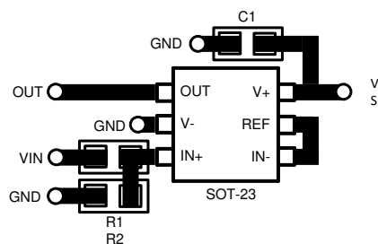
10-7. Layout Example
