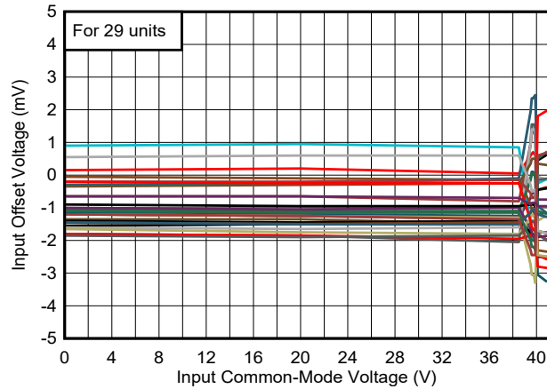
図 6-7. Offset vs. Common-Mode, 40 V
