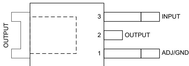
図 4-4. KVV パッケージ、3 ピン TO-252 (上面図)
