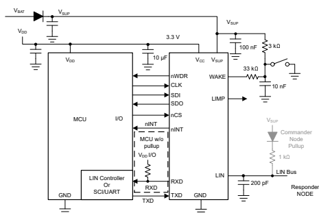
概略回路図、SPI モード
