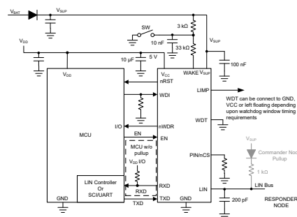
概略回路図、ピン・モード
