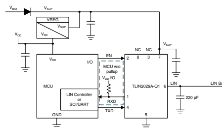
概略回路図、レスポンダモード
