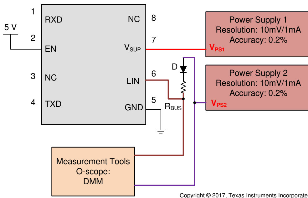
図 6-5. V_SUP_NON_OP Param 11
