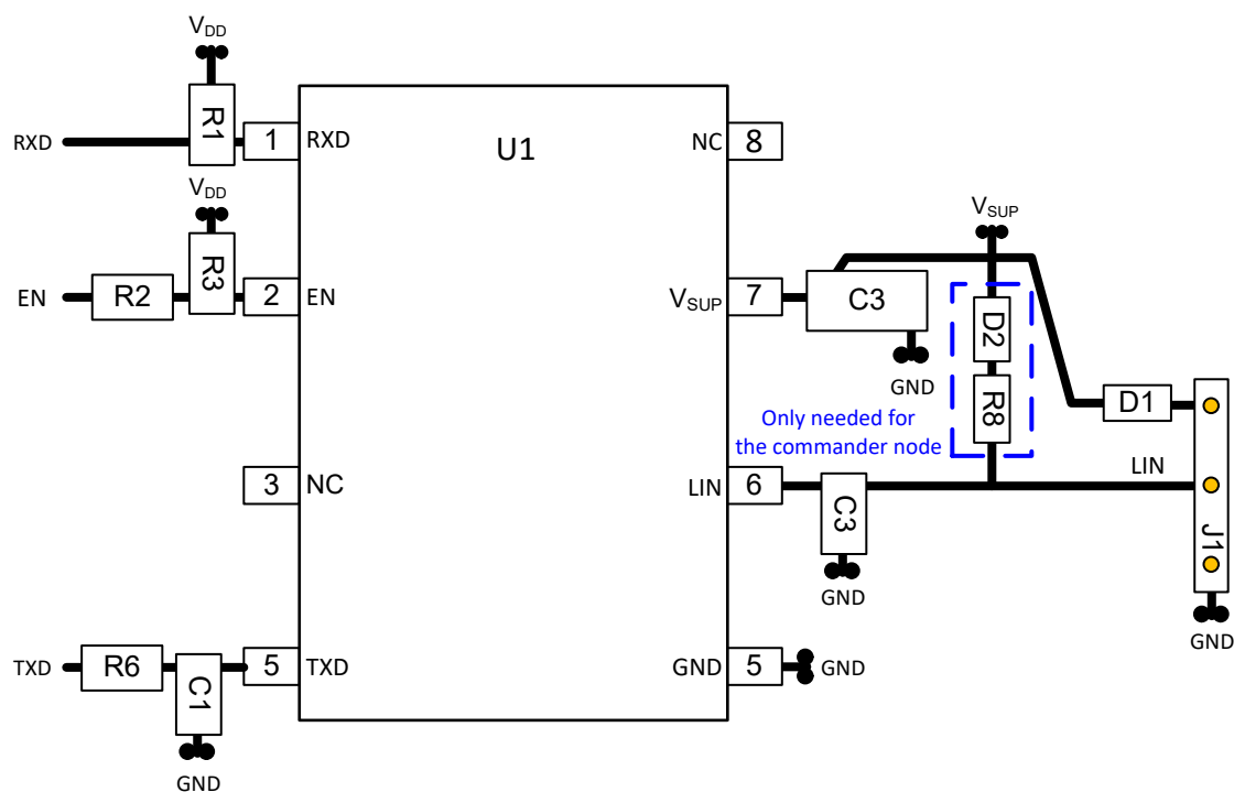
图 12-1. Layout Example
