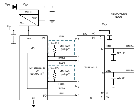
概略回路図、レスポンス・モード
