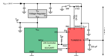
レスポンド・ノードの概略回路図
