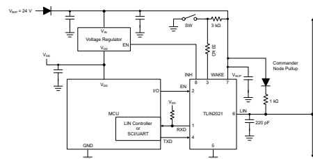
コマンド・ノードの概略回路図
