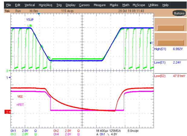
10-9. TLIN1028S-Q1 Brownout
