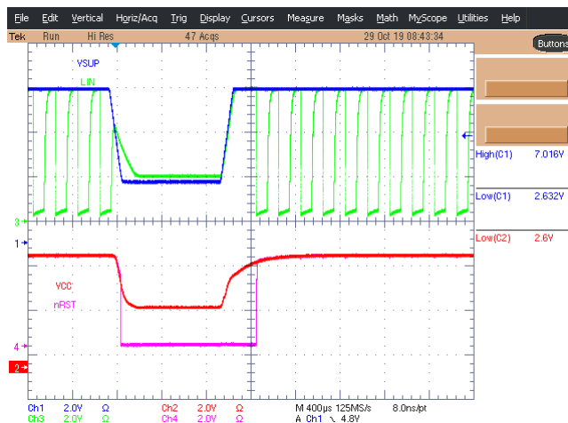
10-18. TLIN10285-Q1 Brownout
