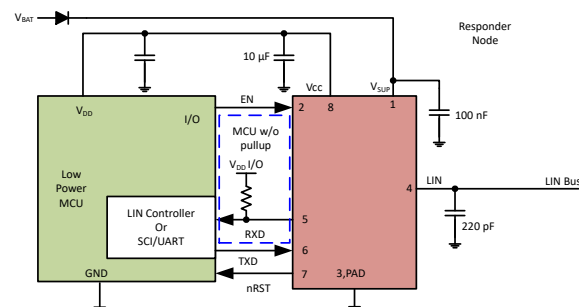
概略回路図、レスポンド・ノード(2)
