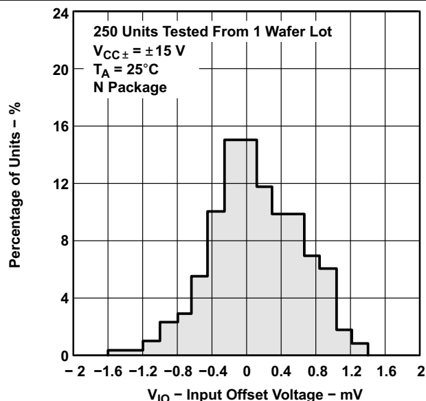
図 5-1. TLE2141 入力オフセット電圧の分布
