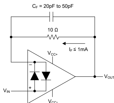
図 7-1. 電圧フォロワ
