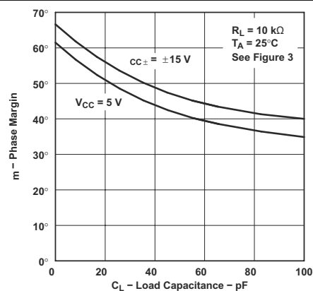
図 6-50. TLE2022 および TLE2024 の位相マージンと負荷容量との関係
