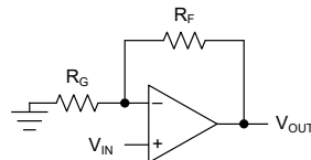
図 7-3. 回路図
