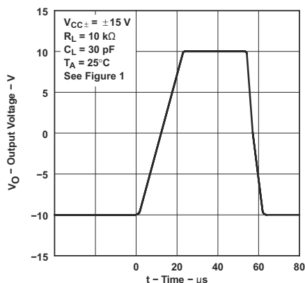
図 5-43. TLE2024-Q1 ボルテージフォロワの大スケールパルス応答
