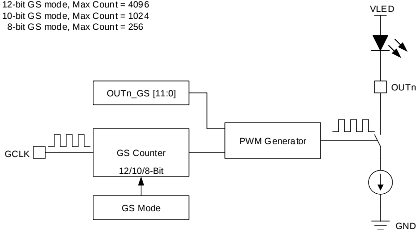
FIG 22. PWM Generator
