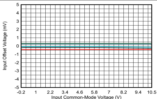
図 6-2. オフセットと同相との関係、12V
