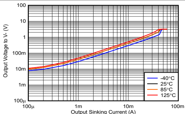
図 6-4. 出力電圧とシンク電流の関係、3.3V
