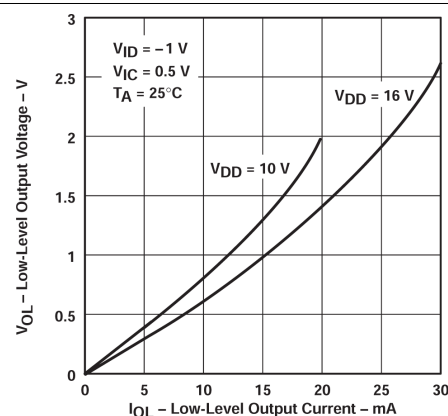
図 5-14. Low レベル出力電圧と Low レベル出力電流との関係
