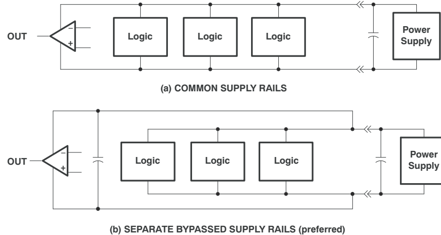
図 7-2. 一般的な電源レールと個別の電源レールの関係
