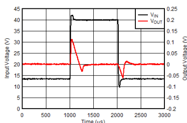
ライン過渡応答 (3V/ \mu s の V_{IN} スループレート) (新しいチップ)
