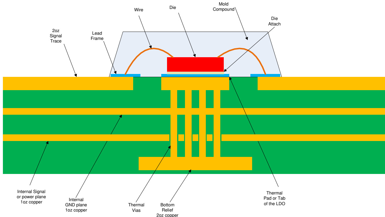
図 8-1. JEDEC Standard 2s2p PCB
