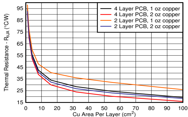
図 8-2. R_{\theta JA} vs Copper Area (KVU Package)
