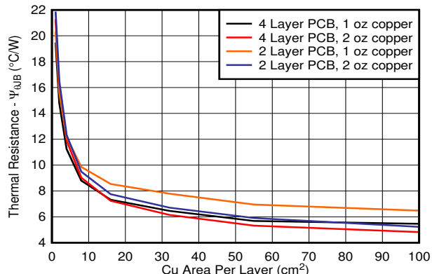
図 8-3. \psi_{JB} vs Copper Area (KVU Package)
