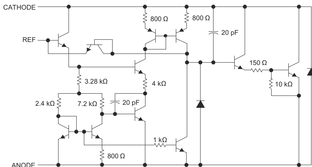
図 8-2. 詳細回路図
