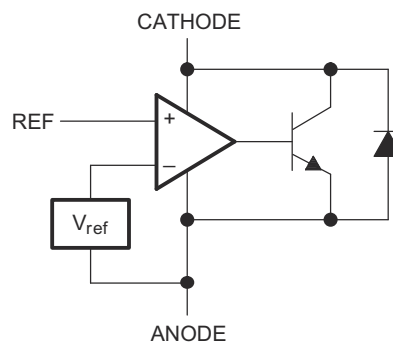
図 8-1. 等価回路図
