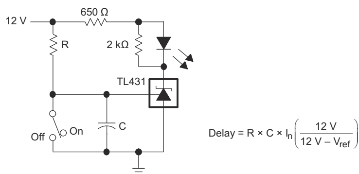
図 9-13. 遅延タイマ
