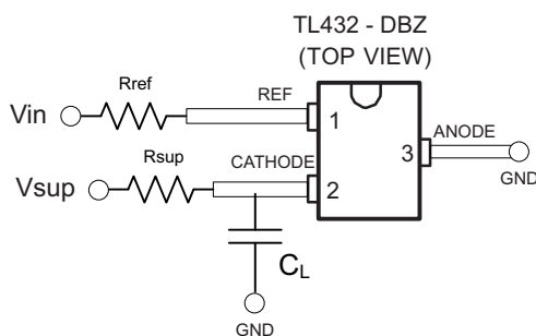
図 9-16. DBZ レイアウト例
