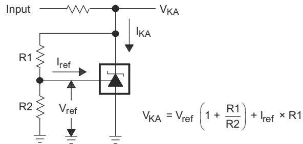
図 7-2. V_{KA} > V_{ref} のテスト回路
